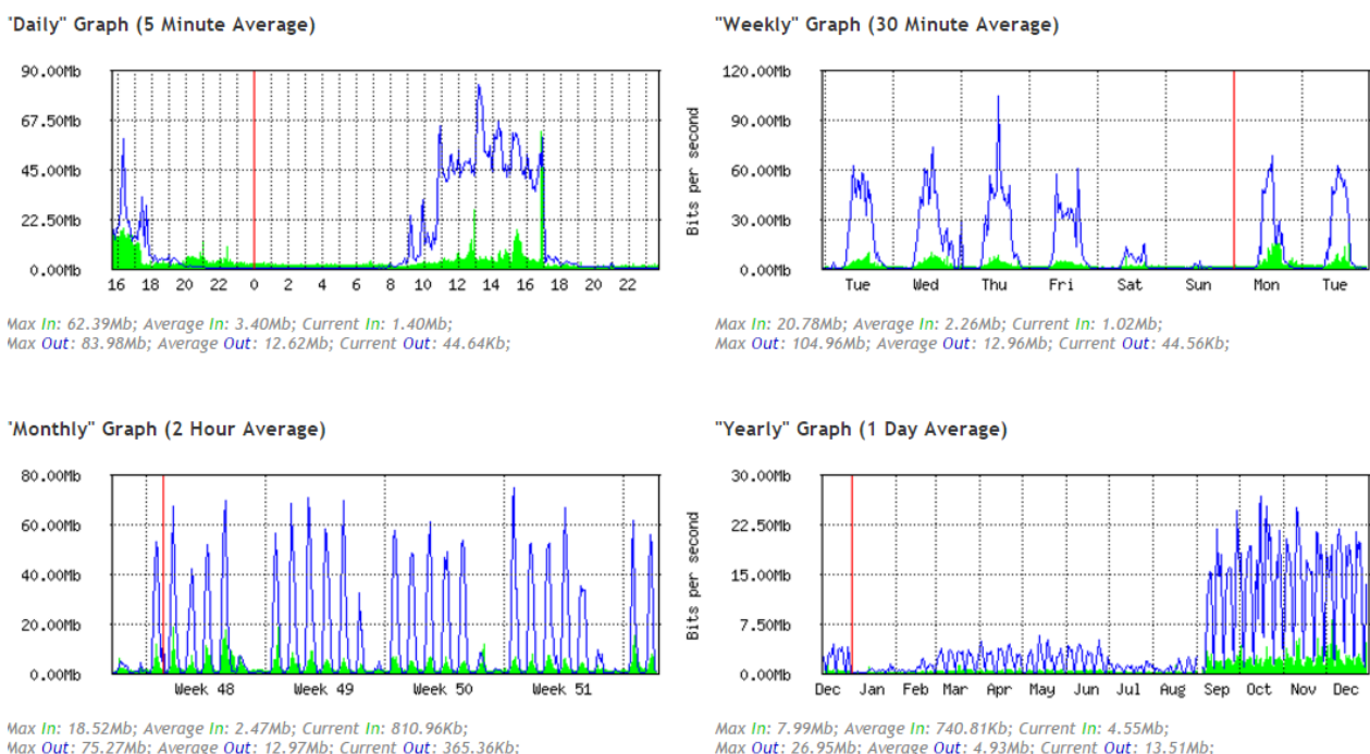
Рис. 25. Завантаженість Інтернет-каналу Центрального корпусу:
